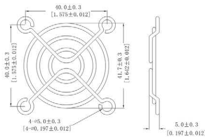
5CM网罩
