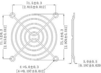
8CM网罩
