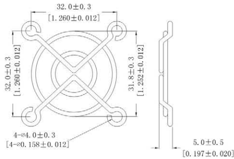
4CM网罩
