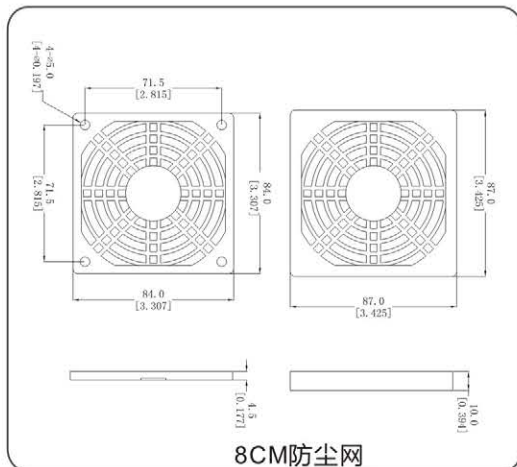
8CM防尘网
