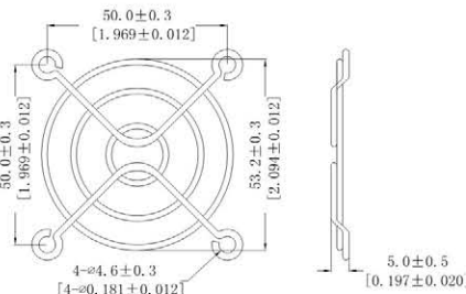
6CM网罩
