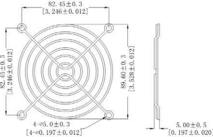
9CM网罩
