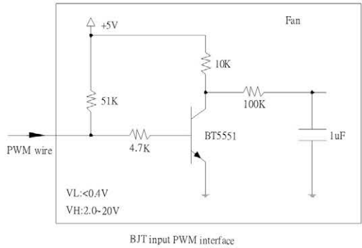
VC(电压讯号调速)输入标准接口电路/VC input standard diagram
