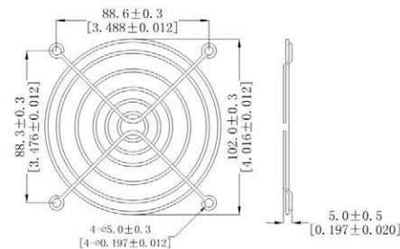
11CM网罩
