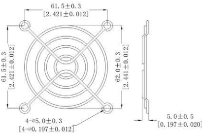
7CM网罩
