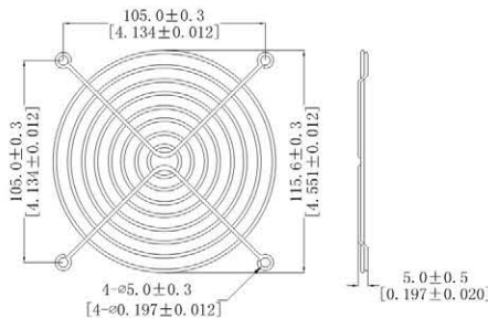
12CM网罩
